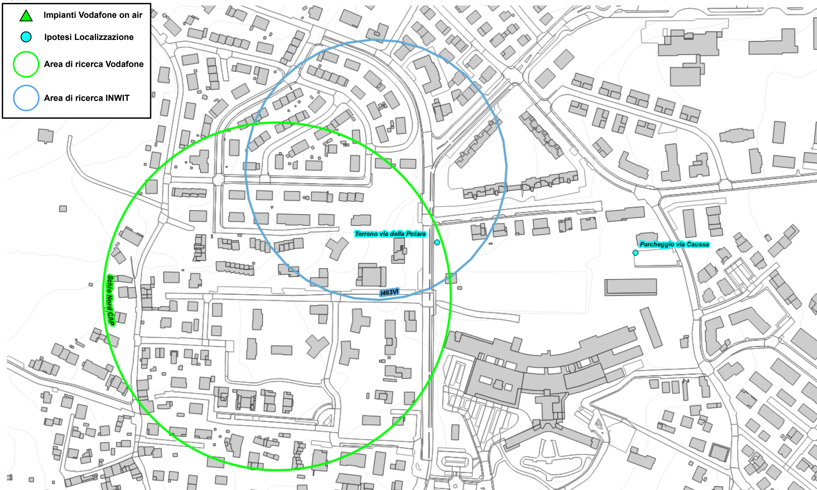
Fig. 25 Dettaglio piano di rete – Gestore VODAFONE
