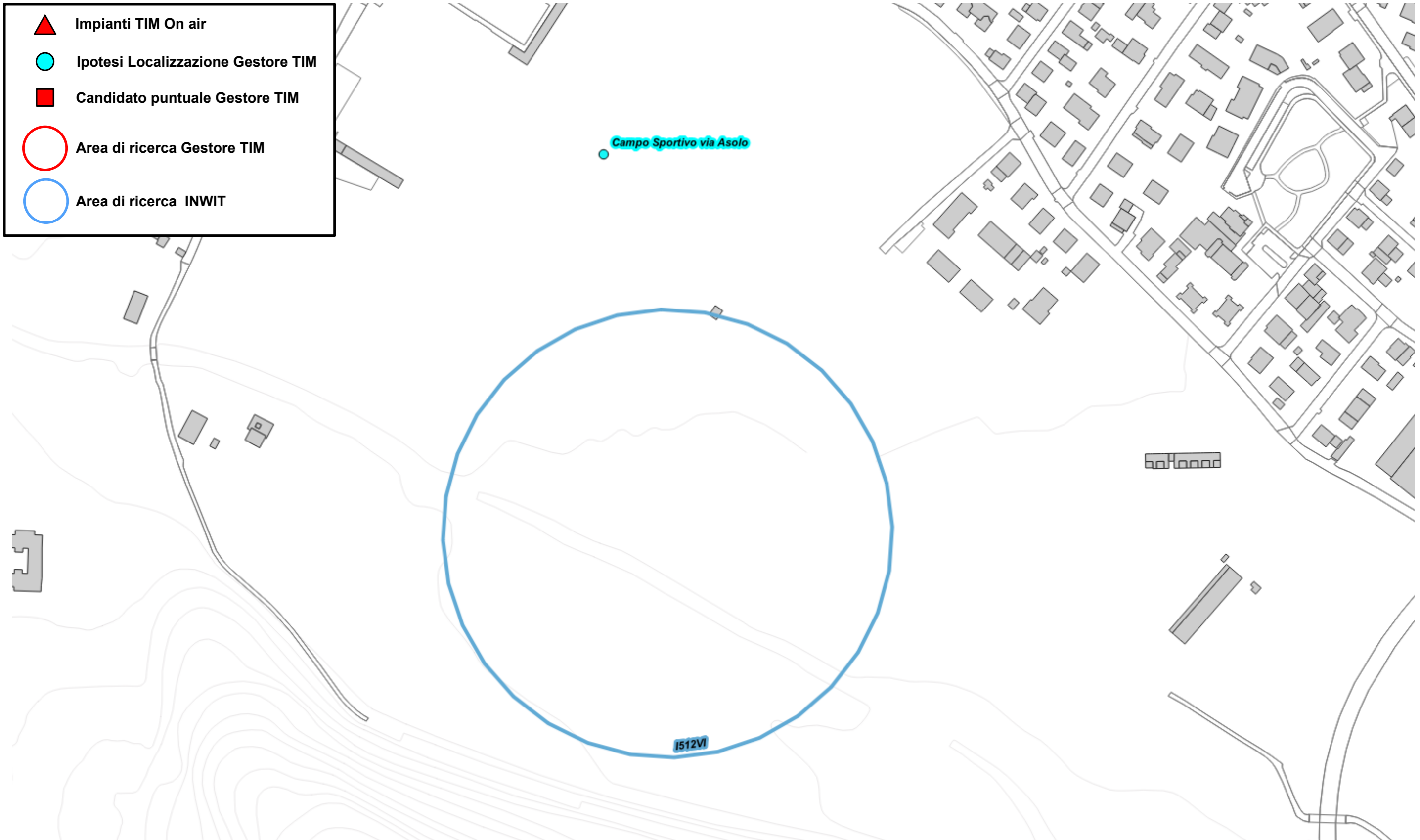
Fig. 22 Dettaglio piano di rete – Gestore TIM
