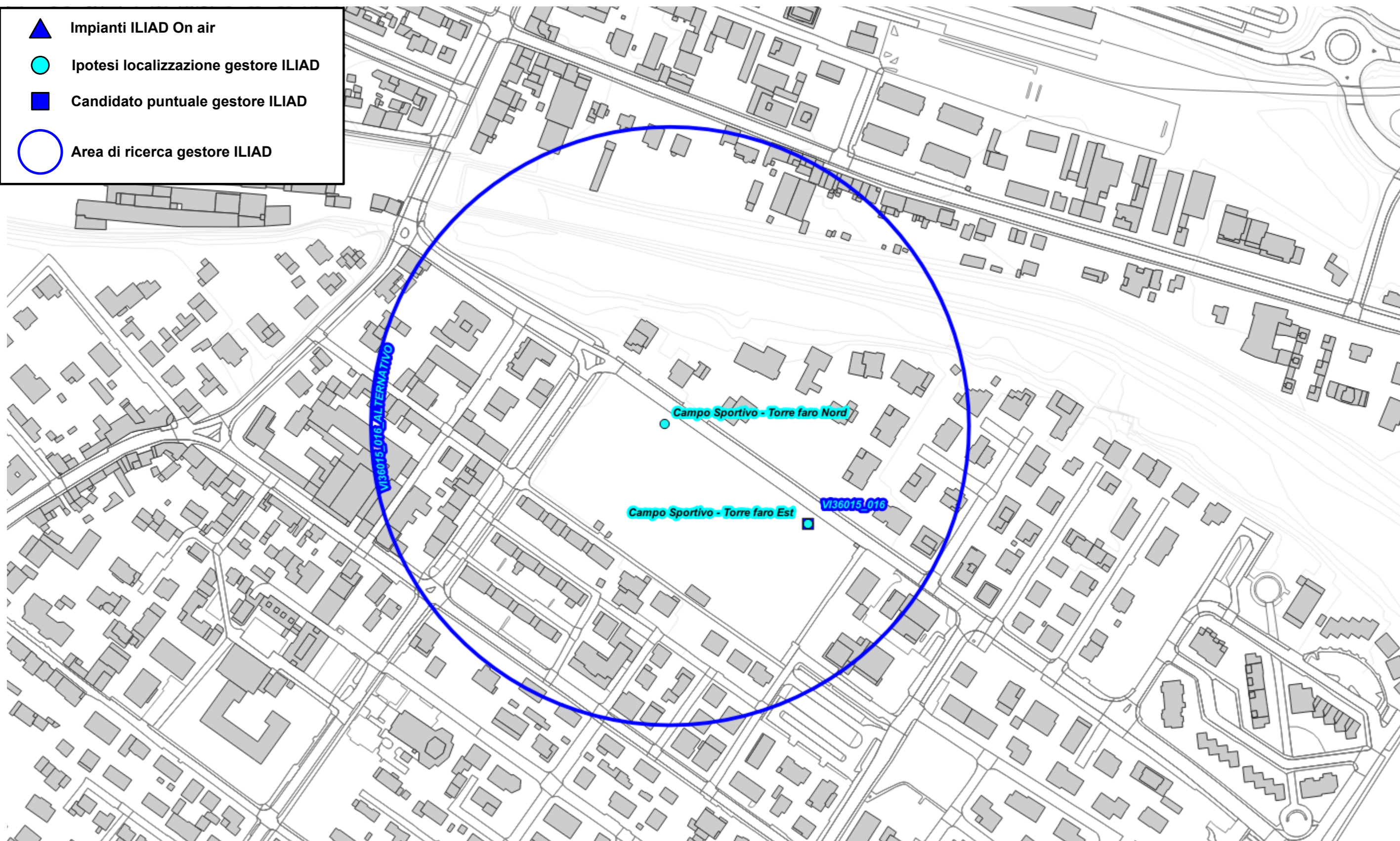
Fig. 39 Dettaglio piano di rete – Gestore ILIAD
