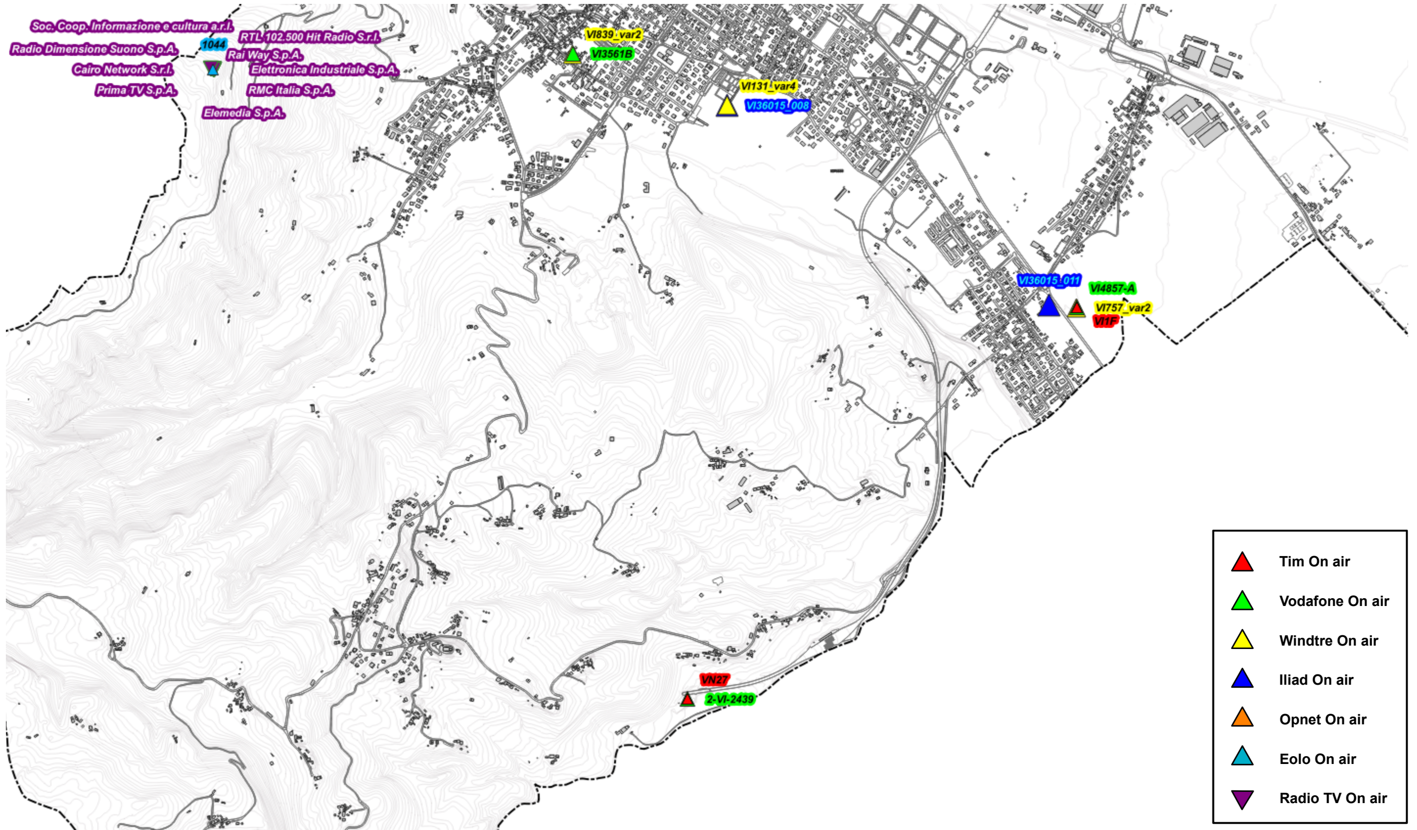
Fig. 11 Dettaglio impianti Onair – Quadro di sintesi
