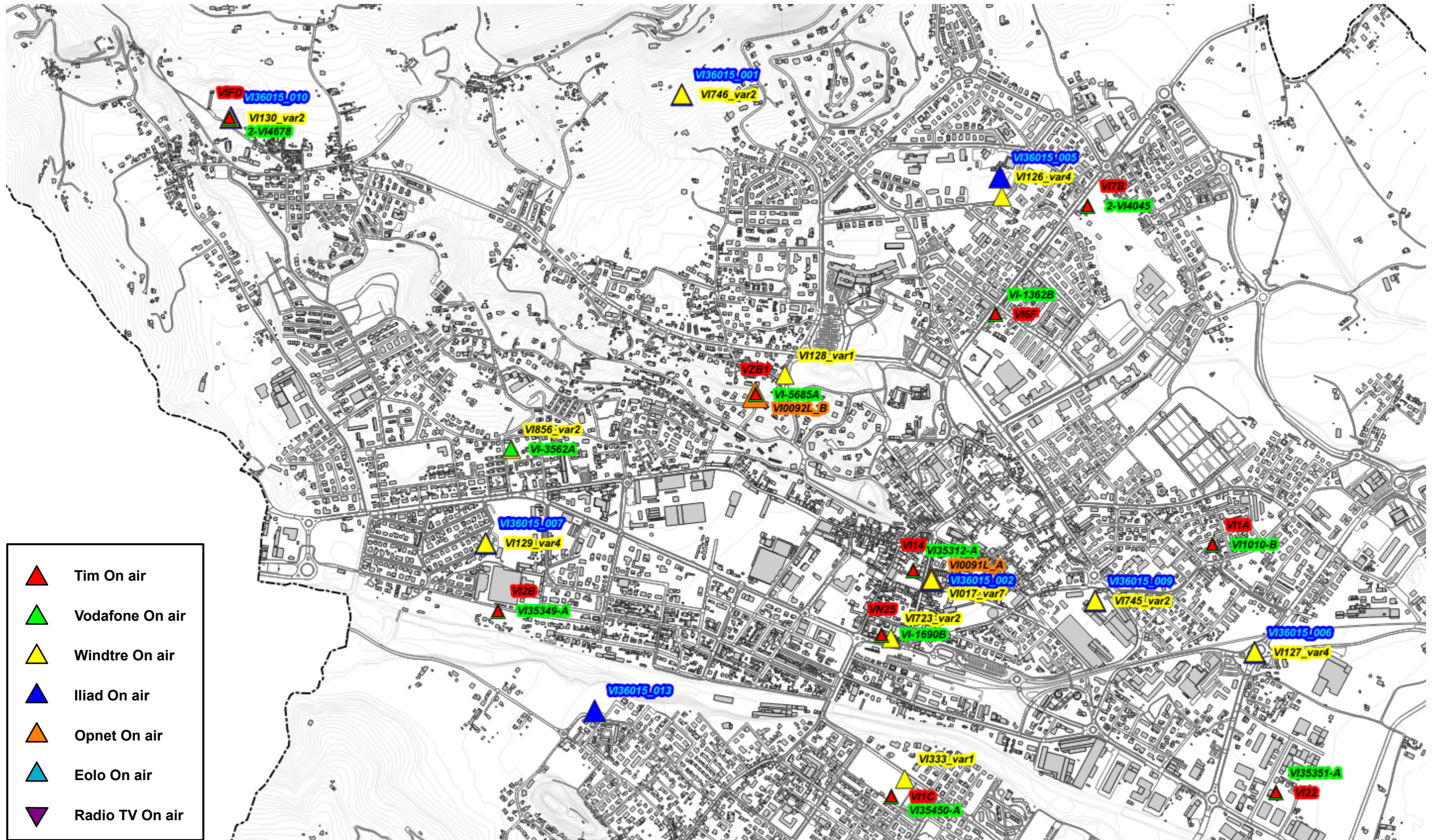
Fig. 9 Dettaglio impianti Onair – Quadro di sintesi
