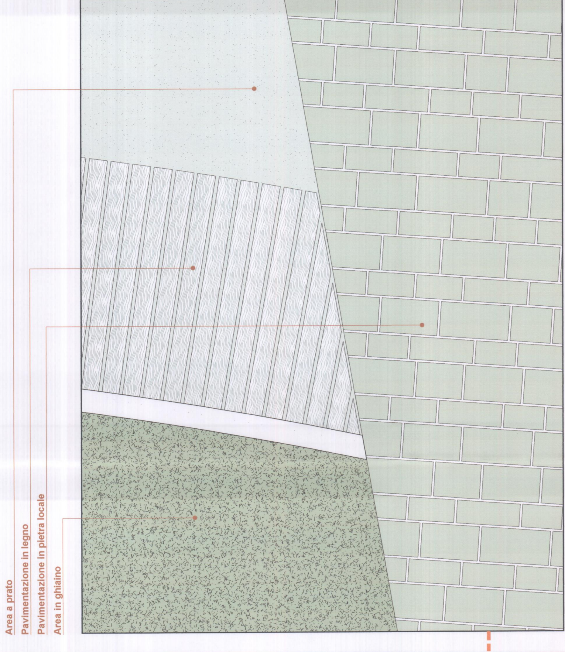
PARTICOLARE 1 - Scala 1:20
